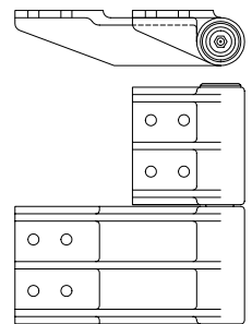
Top Hinge for L.H. Door
