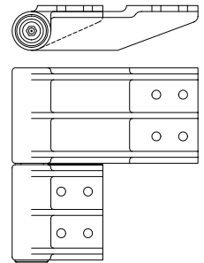
Bottom Hinge for R.H. Door
