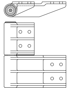
Top Hinge for R.H. Door
