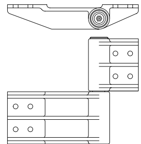
Top Hinge for L.H. Door
