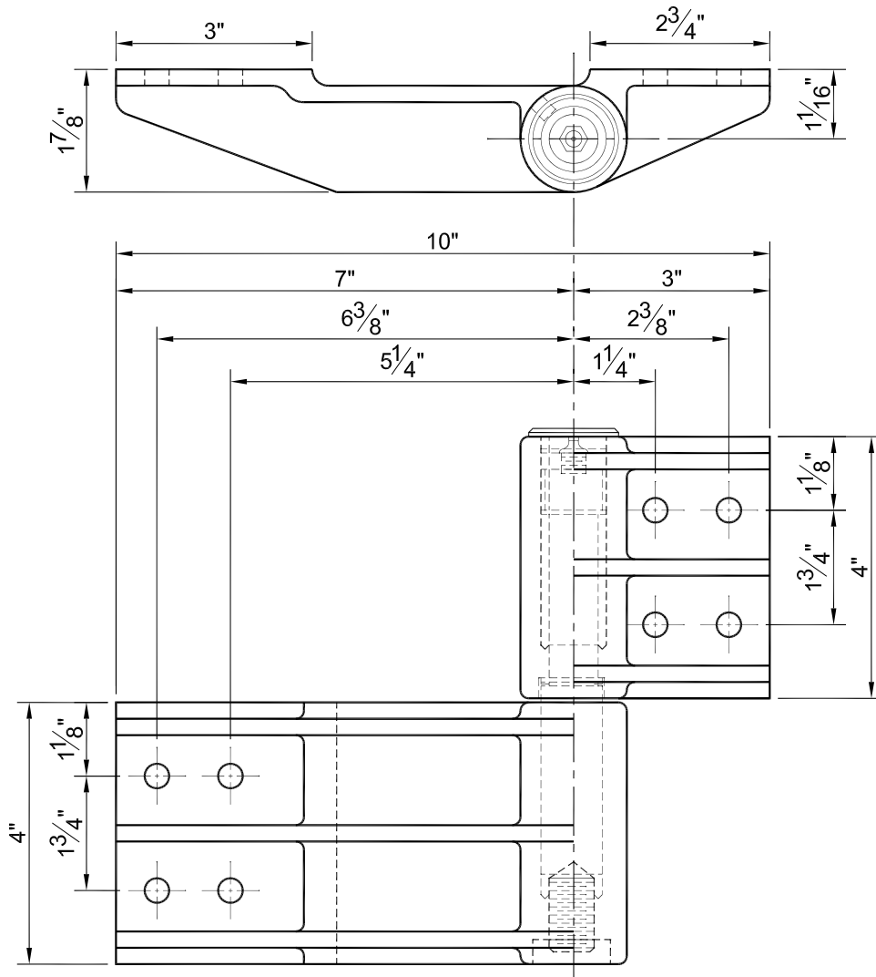
Type S-1800 Hinge Top Hinge for L.H. Door
