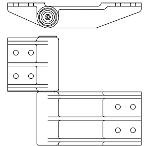
Top Hinge for R.H. Door
