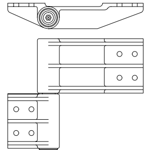
Bottom Hinge for R.H. Door
