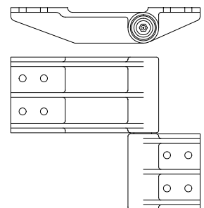
Bottom Hinge for L.H. Door
